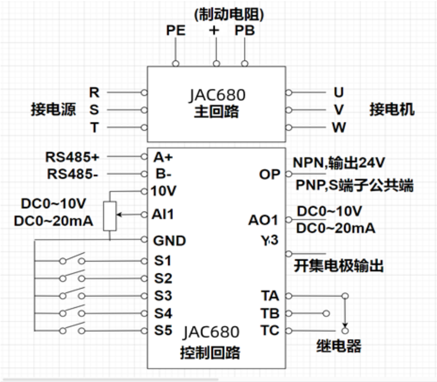
变频器控制端子功能说明：
